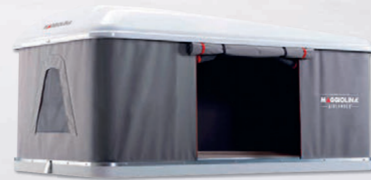
Hartschalendachzelt AIRLANDER Per Kurbel wird die Oberschale angehoben und der Zeltstoff gespannt. So entsteht ein 210 cm x 145 cm großer Schlafplatz mit integriertem Moskitonetz.
