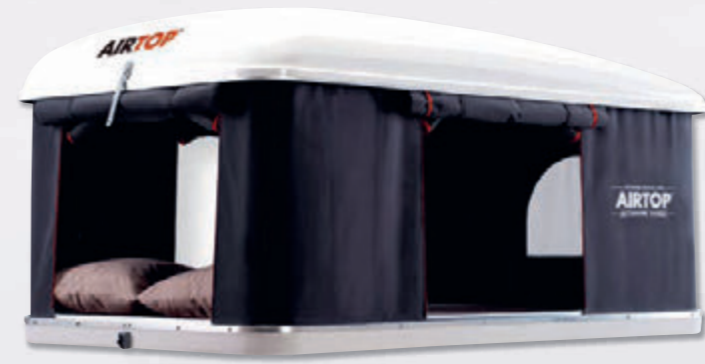
Hartschalendachzelt AIRTOP Vier Gasdruckfedern heben die Oberschale und das durch ein Moskitonetz geschützte 210 cm x 145 cm große Dachapartment ist einsatzbereit.
